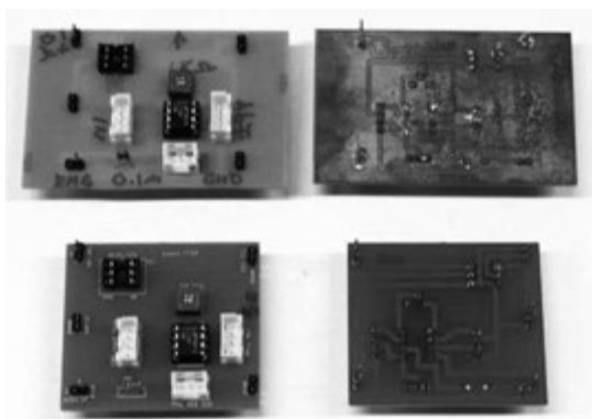
図4. 銅張積層板(上段)とプリント基板(下段)
