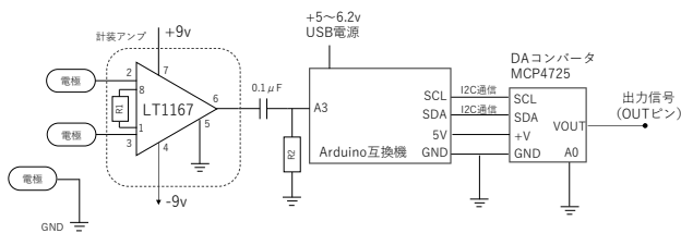
図 2. 筋電図スイッチ回路図
